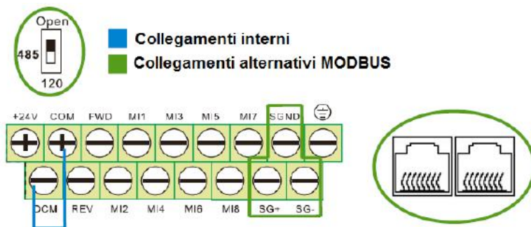
FIGURA 20: collegamento RS485
