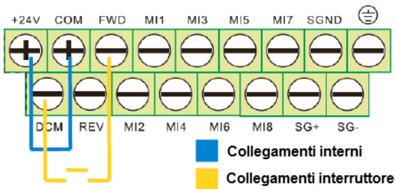
FIGURA 10: azionamento automatico interruttore/PLC – collegamento NPN
